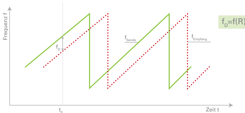
Bild 2: Zeitabhängiger Verlauf der Sende- und Empfangsfrequenzen beim FMCW-Radar mit Sägezahnmodulation
