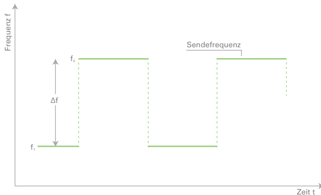
Abb 3: Grundsätzlicher Zeitverlauf der Sendefrequenz bei einem FSK-Radar nach dem Frequenzsprungverfahren
