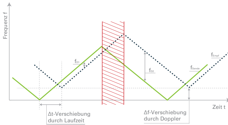
Bild 4: Zeitlicher Verlauf von Sende- und Empfangsfrequenzen beim FMCW-Radar mit Dreiecksmodulation
