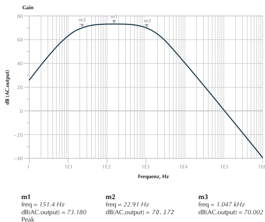
Bild 7: Vorschlag Nachverstärkerschaltung für einen Kanal, Verstärkung 70dB, 1 kHz Bandbreite
