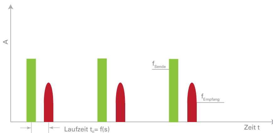
Bild 1: zeitlicher Verlauf von Sende- und Empfangsimpuls bei einem Pulsradar
