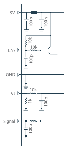
Bild 9: Interface und interne Beschaltung von InnoSenT Radarmodulen, insbesondere von IVS-148
