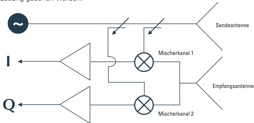
Bild 5: Prinzipschaltbild eines InnoSenT-Radarfrontends mit getrennten Sende/Empfangsantennen.
