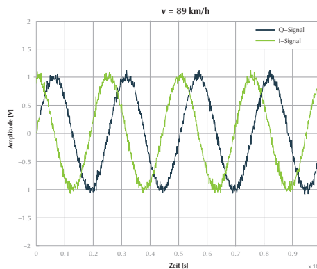
Bild 6: Typisches Scope-Bild der beiden I/Q-Ausgänge eines Radarsensors bei einem gleichförmig bewegten Ziel
