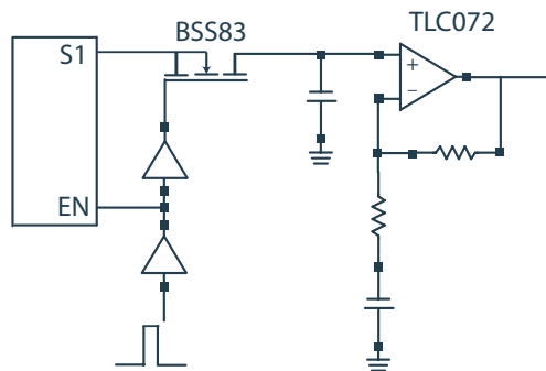
Bild 8: Getakteter Radarsensor mit Sample & Hold – Schaltung
